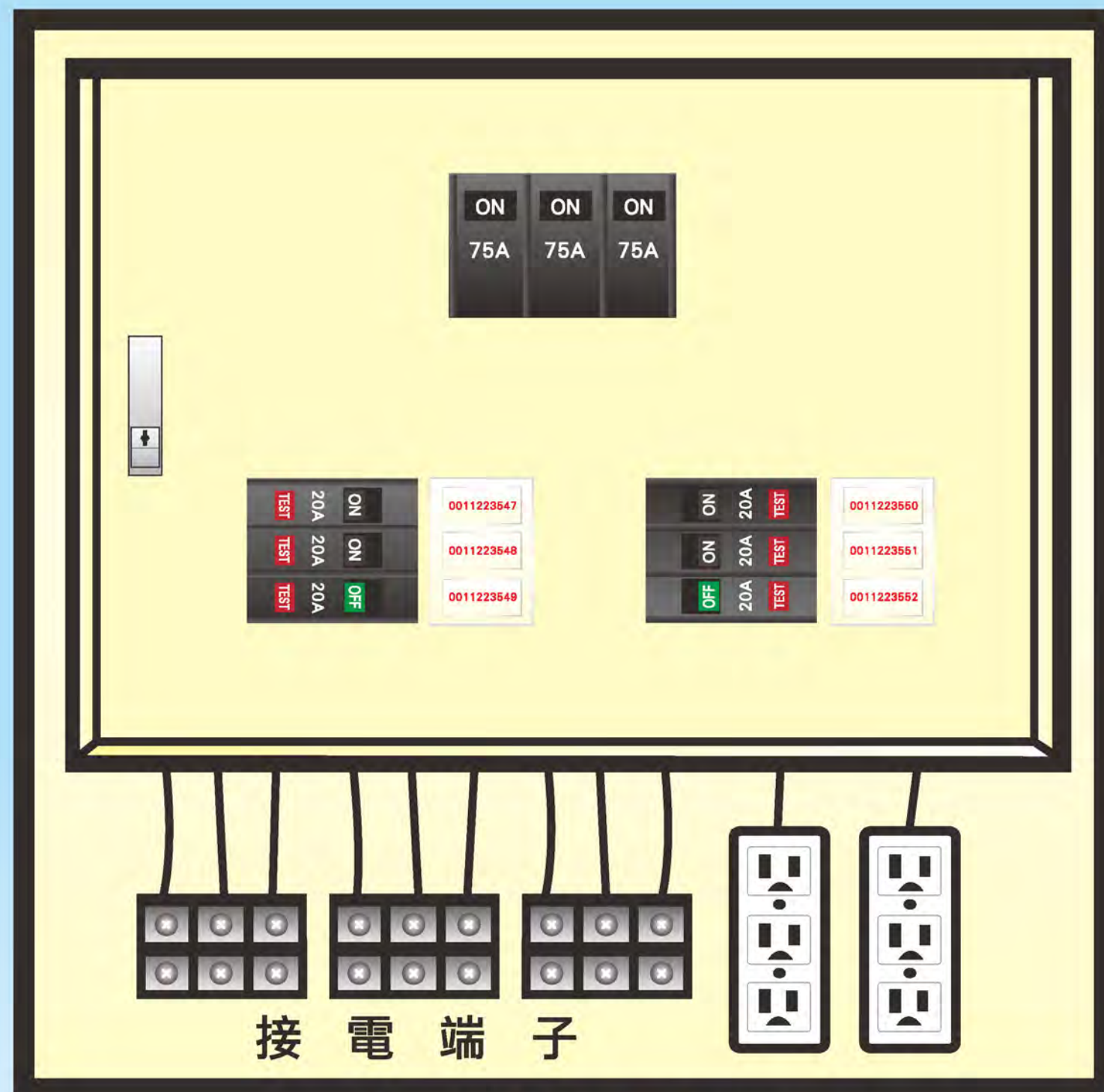
配電箱內部圖
