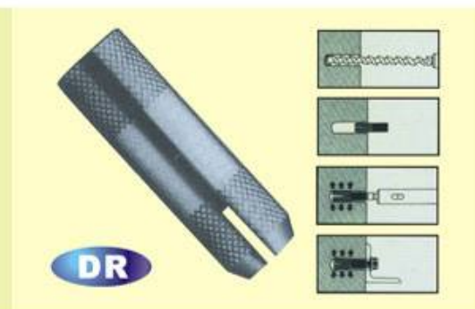
內迫式膨脹螺絲 DROPIN ANCHOR
