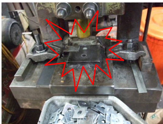
說明：現場衝床未設置安全護圍。
