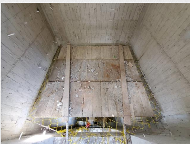
電梯井開口應設置護欄、 護蓋或安全網等防護設備
